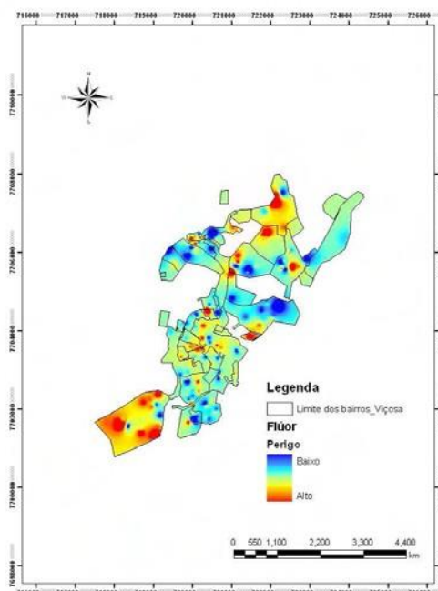
d) Flúor – mg/L
