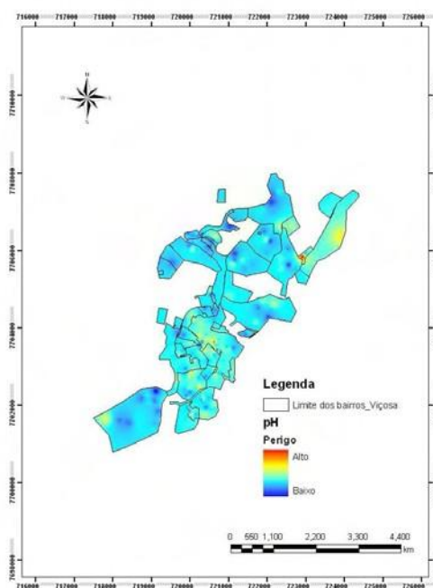
f) pH - unidades de pH
